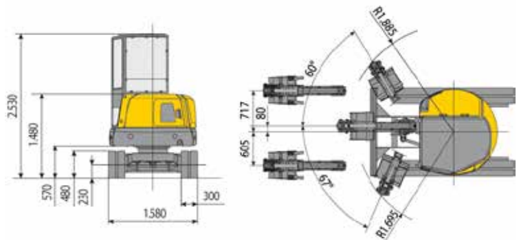
Balancier standard (Balancier en option)
